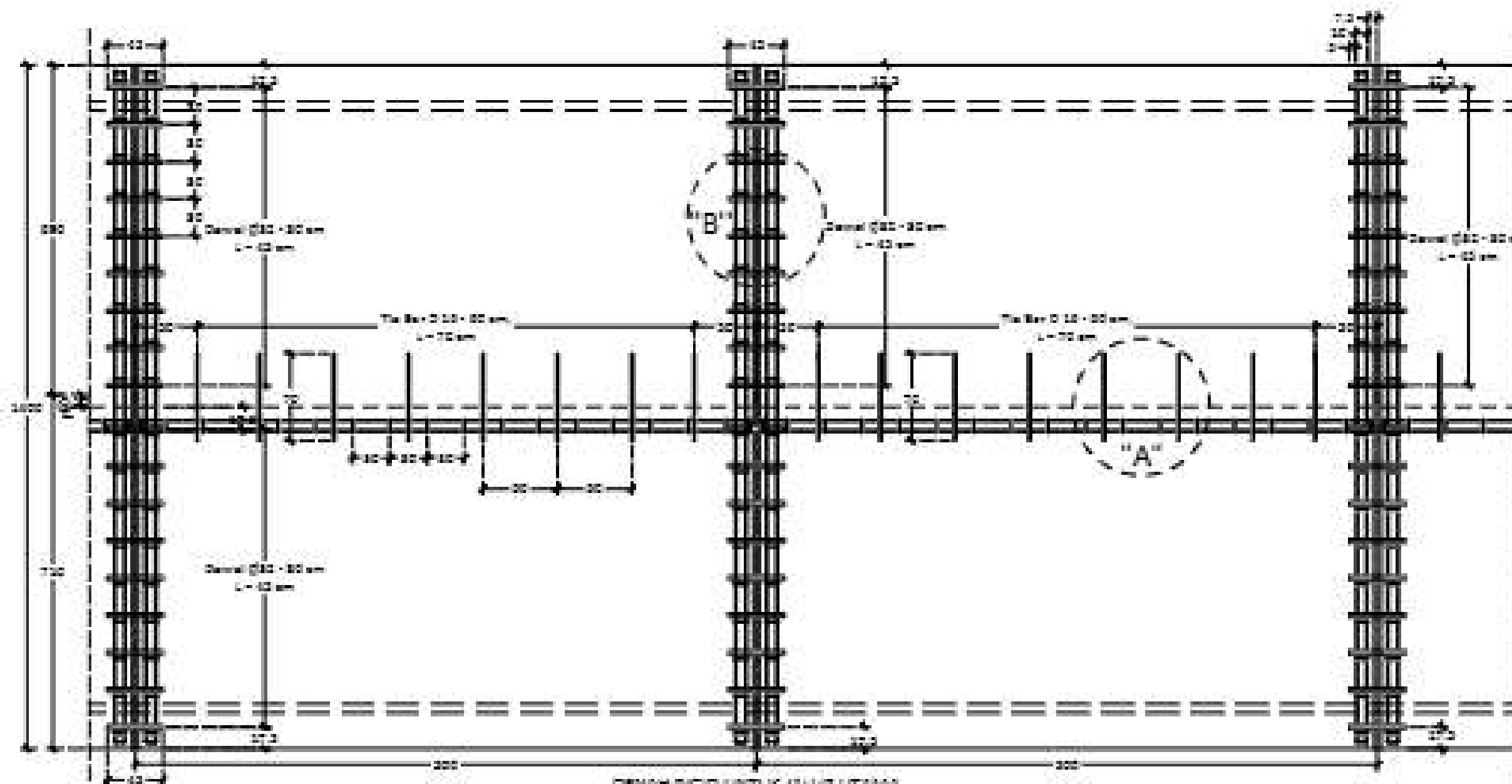
DENAH RIGID UNTUK JALUR UTAMA
